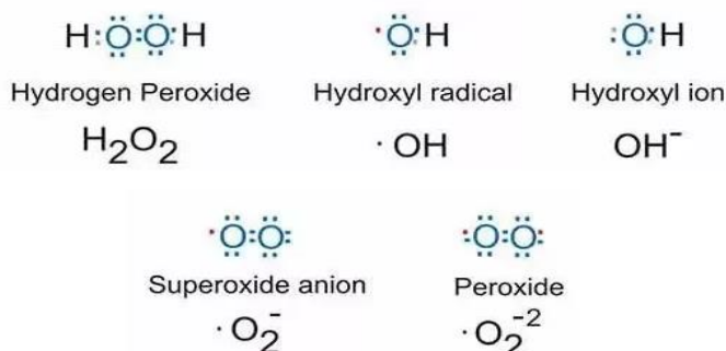
شکل ۱۱- ساختار مولکولی تعدادی از گونه های فعال اکسیژن. هیدروژن پروکسید و یون هیدروکسیل گونه فعال غیر رادیکالی و سه گونه دیگر رادیکال هستند (Chaudhary et al., 2023)
