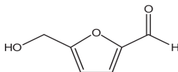
شکل ۱۴ - ساختار هیدروکسی متیل فورفورال (HMF) (Shapla et al., 2018)
