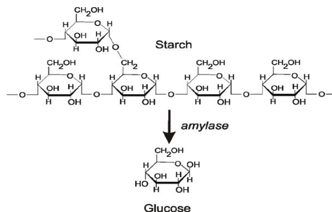
شکل ۵- تبدیل نشاسته به واحدهای گلوکز توسط آمیلاز (Alaerjani et al. , 2022)
