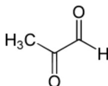
شکل ۱۶- فرمول متیل گلی اکسال (Alvarez-Suarez et al. , 2014)
