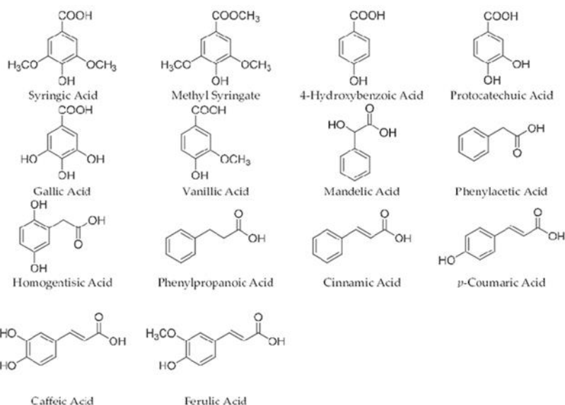
شکل ۳- ساختار مولکولی اسیدهای فنلی با تک حلقه آروماتیک در عسل (Liu et al. , 2020) Fig. 3- Molecular structure of phenolic acids with a single aromatic ring in honey (Liu et al. , 2020)
