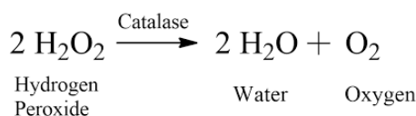
شکل ۷ - واکنش تبدیل آب اکسیژنه (H 2 O 2 ) به آب و اکسیژن توسط کاتالاز (Alshareef et al., 2022) Fig. 7- Conversion of hydrogen peroxide (H 2 O 2 ) into water and oxygen by catalase (Alshareef et al., 2022)
