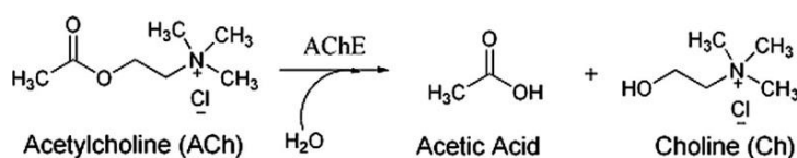
شکل ۸- واکنش تبدیل استیل کولین به استیک اسید و کولین توسط استیل کولین استراز (AChE) (Tōugu, 2001) Fig. 8- Conversion of acetylcholine to acetic acid and choline by acetylcholinesterase (AChE) (Tōugu, 2001)
