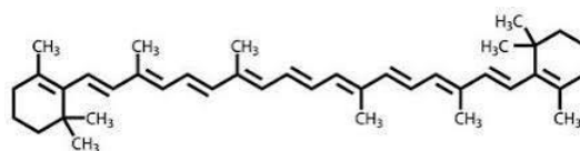
شکل ۱۲- ساختار بتا کاروتن (Ranneh et al. , 2021)
