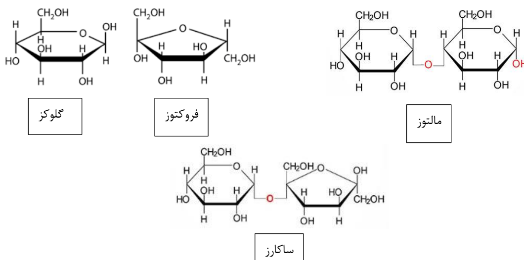
شکل ۱- ساختار حلقوی برخی از قندهای عسل، گلوکز و فروکتوز تک قندی های احیا کننده، مالتوز دوقندی احیا کننده و ساکارز دوقندی غیر احیا کننده (Tafere, 2021)
