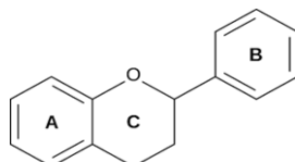
شکل ۹- ساختار پایه فلاونوئیدها (حلقه فلاوان) (Cianciosi et al. , 2018) Fig. 9- Basic structure of flavonoids (flavan ring) (Cianciosi et al. , 2018)
