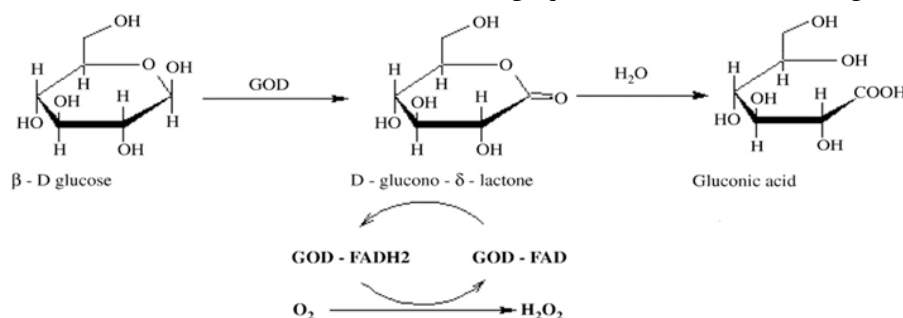
شکل ۶ - واکنش تبدیل گلوکز به اسید گلوکونیک و آب اکسیژنه توسط آنزیم گلوکز اکسیداز (Wang et al., 2022) Fig. 6- Conversion of glucose into gluconic acid and hydrogen peroxide by the enzyme glucose oxidase (Wang et al., 2022)
