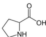
شکل ۲- ساختار پرولین (Carter et al 2006) Fig. 2- Proline structure (Carter et al 2006)
