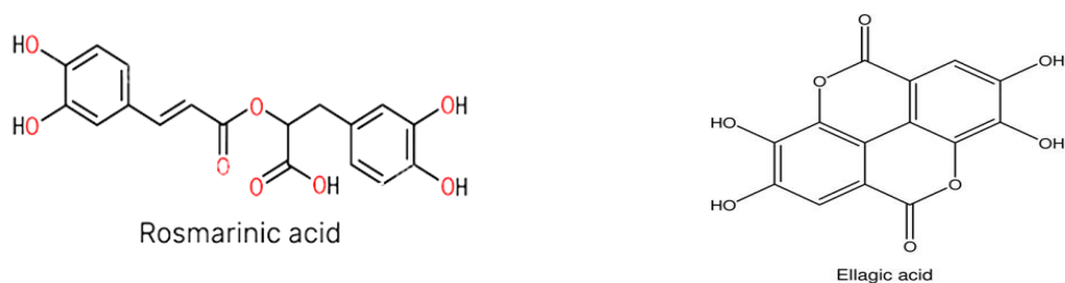
شکل ۴- ساختار مولکولی اسیدهای چند فنلی با چند حلقه آروماتیک در عسل (Liu et al. , 2020) Fig. 4- Molecular structure of polyphenolic acids with multiple aromatic rings in honey (Liu et al. , 2020)
