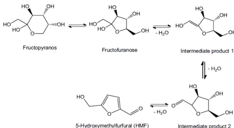
شکل ۱۵- چگونگی تبدیل قند فروکتوز ( اینجا به شکل فروکتوپیرانوز) به هیدروکسی متیل فورفورال (Shapla et al., 2018)
