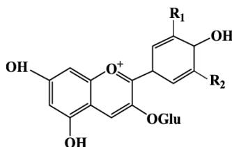
شکل ۱۳ - ساختار مولکولی آنتوسیانین (Ranneh et al. , 2021)
