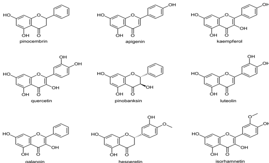
شکل ۱۰- ساختار مولکولی برخی از فلاونوئیدهای عسل. این ترکیبات دارای حلقه های A, B و C فلاوان می باشند و تفاوت آنها در استخلاف های روی حلقه ها می باشد (Panche 2016)
